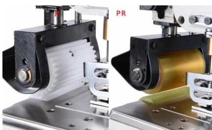
2 rodzaje pullerów dociskowych zapewniają idealne warunki pracy dla zróżnicowanych materiałów
