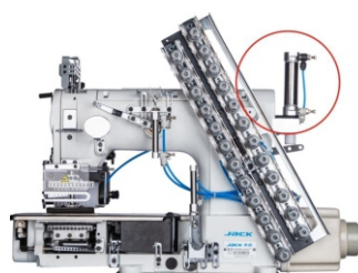
UTL – wersje maszyn z automatycznym obcinaniem nici i podnoszeniem stopki
